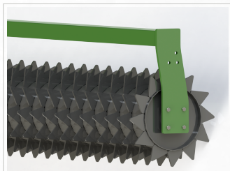
VÁLEC PACKERA
