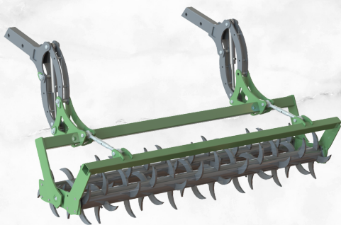
Hrotový válec tandem s hydraulickou regulací
